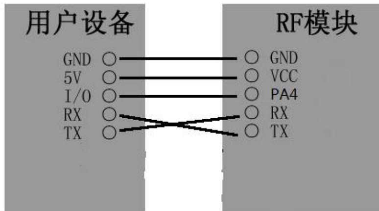
6.1 无线模块和用户设备连接示意图（TTL）
