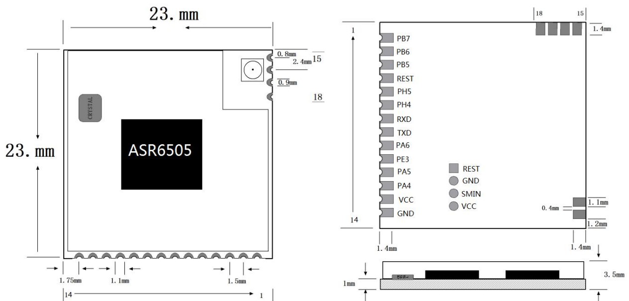
图 4.1 尺寸结构图 ( 单位:mm )
